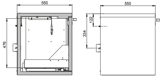
Draufsicht
