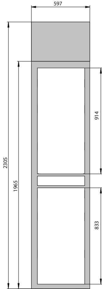
Frontalansicht
