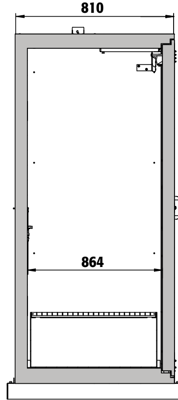
Seitenansicht
