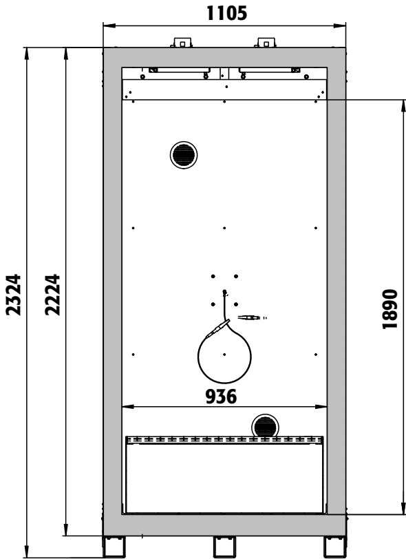
Frontalansicht
