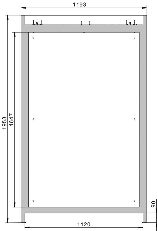
Frontalansicht
